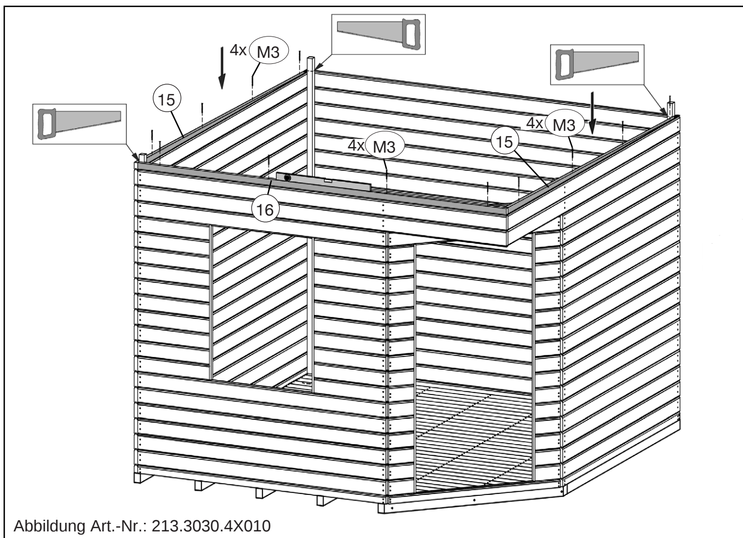
Abb.: Ausrichtung des Gefälles, Richtung des Gefälles durch die Anordnung der oberen Abschlussbohlen variabel! Bei der zusätzlichen Montage eines Anbaus Richtung des Gefälles des Anbaus beachten! (siehe Grafik oben)
