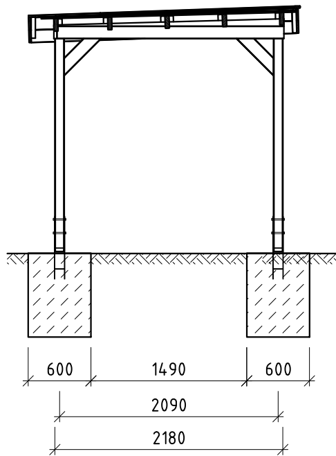
Schnitt A-A M1:50
