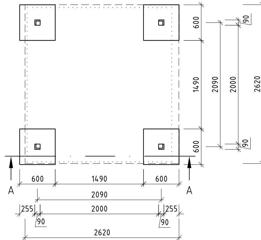
Grundriss
