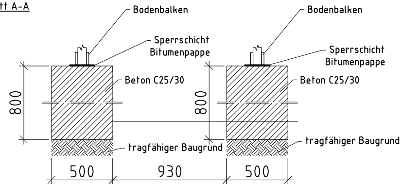
Schnitt A-A
