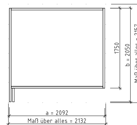
Grundriss M 1:50
