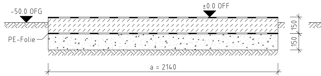
Schnitt A-A M 1:20
