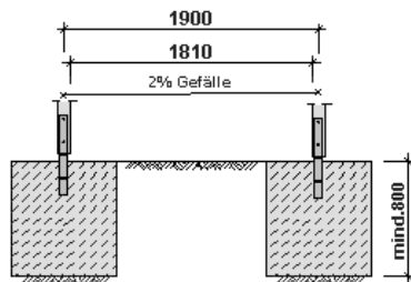
Schnitt B
