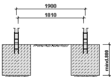
Schnitt B
