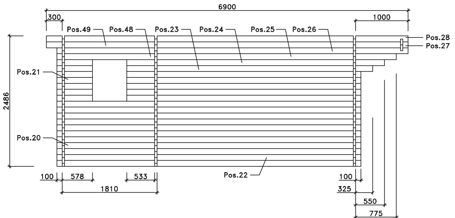
Seitenwand, links
