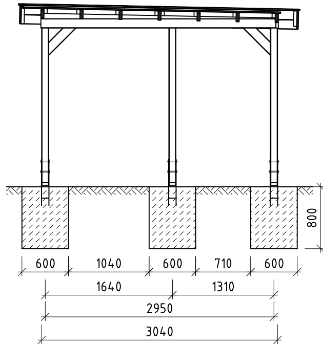
Schnitt A-A M1:50
