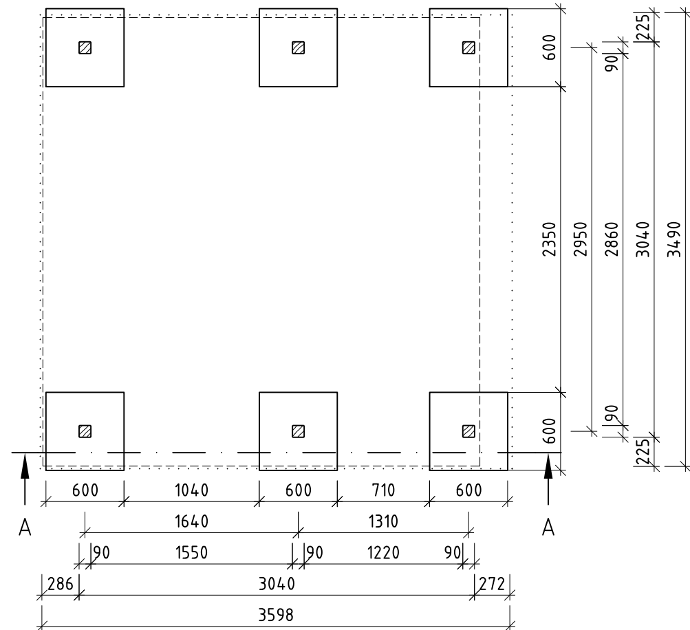
Grundriss
