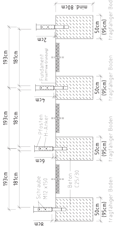
Schnitt B-B
