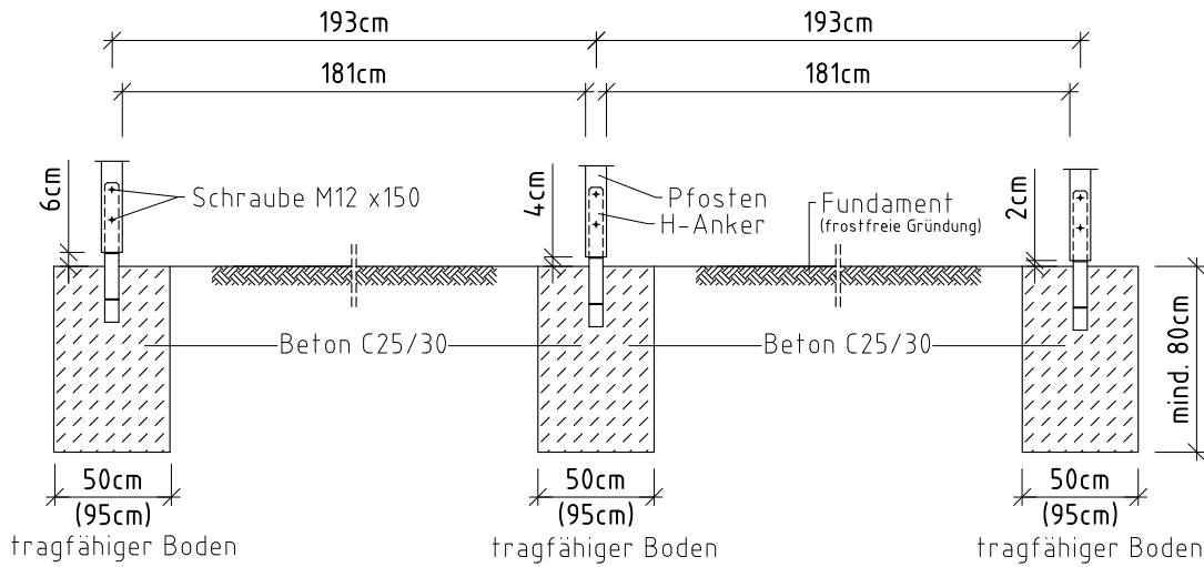
Schnitt B-B
